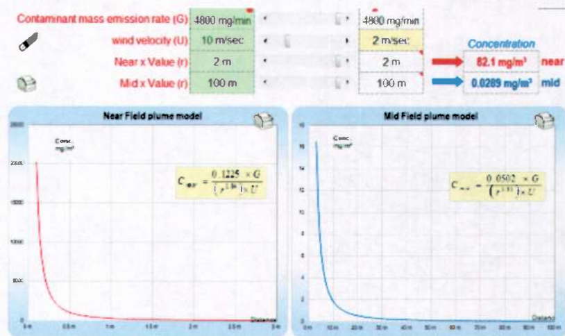
Figur 10: Modellering av spredning av brennerøyk hhv. 2 og 100 m fra brennstedet – kildestyrke 80 mg/s.
